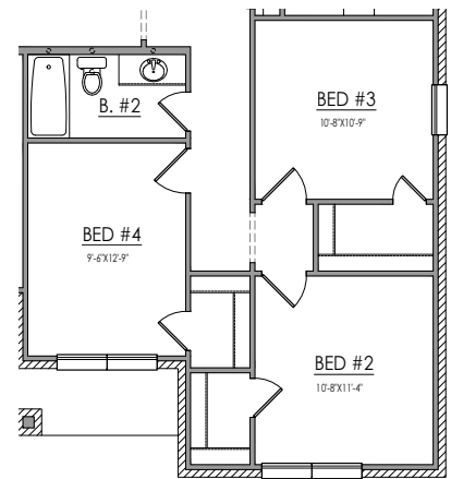
OPTIONAL BED 4 (IN LIEU OF GAME ROOM)
